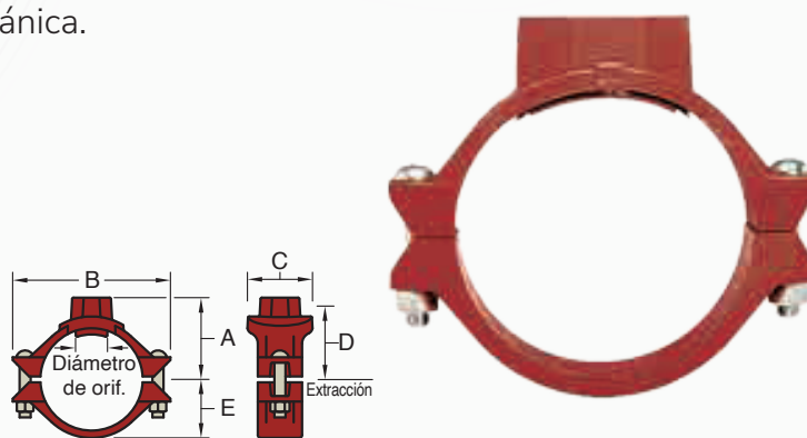
Figura 730 Salida de ramal con ramal roscado hembra BSP (Configuración de té)
